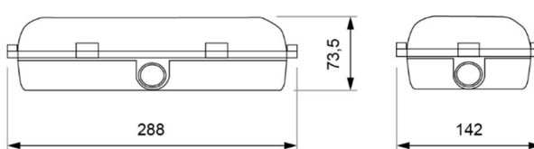
Montaje estanco
